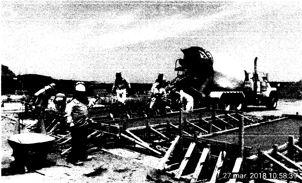
Imagen N°5: A la vista de la imagen se aprecia a los trabajadores realizando trabajos de vaciado de concreto para construir las losas prefabricadas de plataforma del cabezo del muelle con su traje Taimos cumpliendo las Normas de Seguridad Salud.
